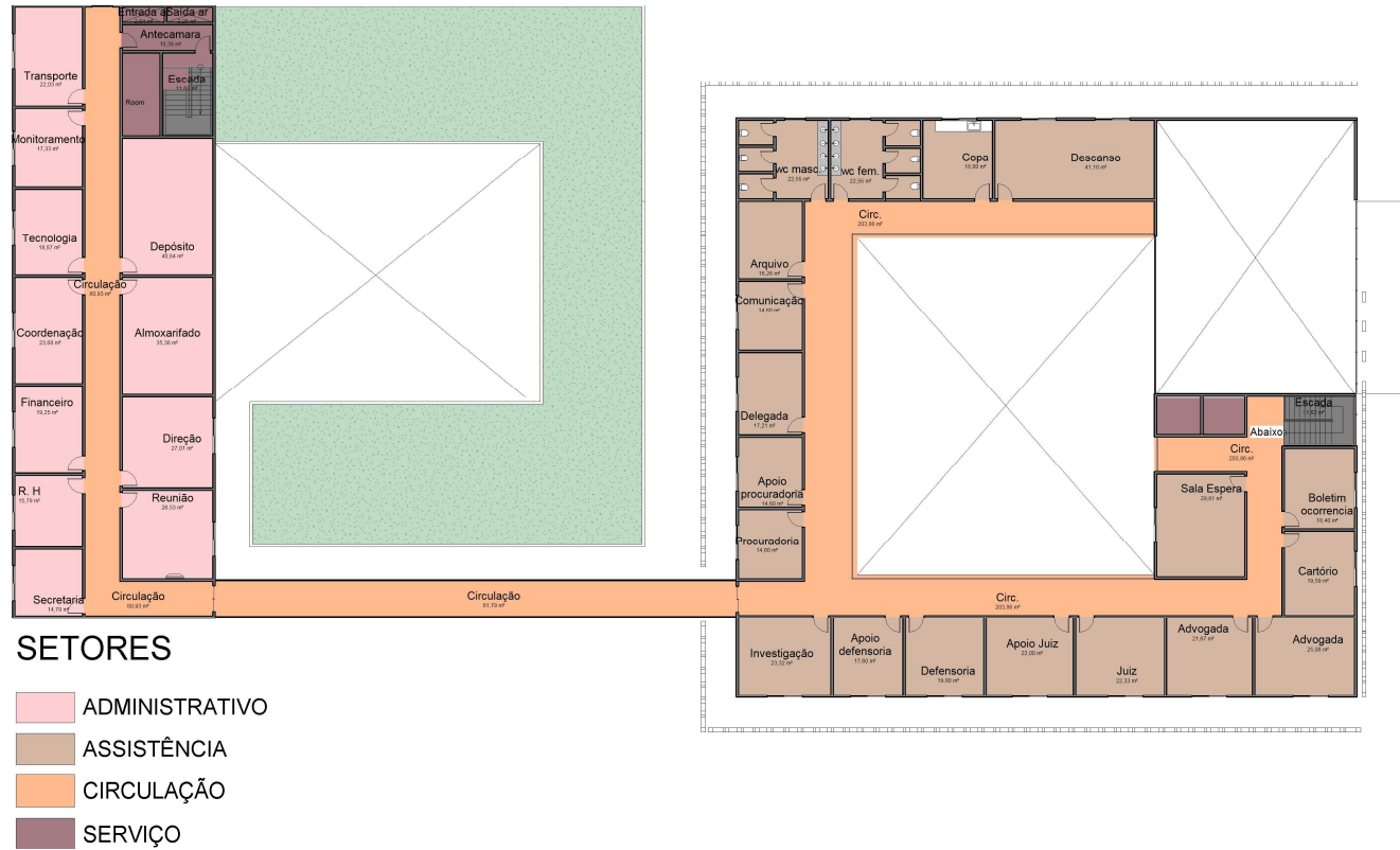
Figura 72 - Setorização Pavimento 1
