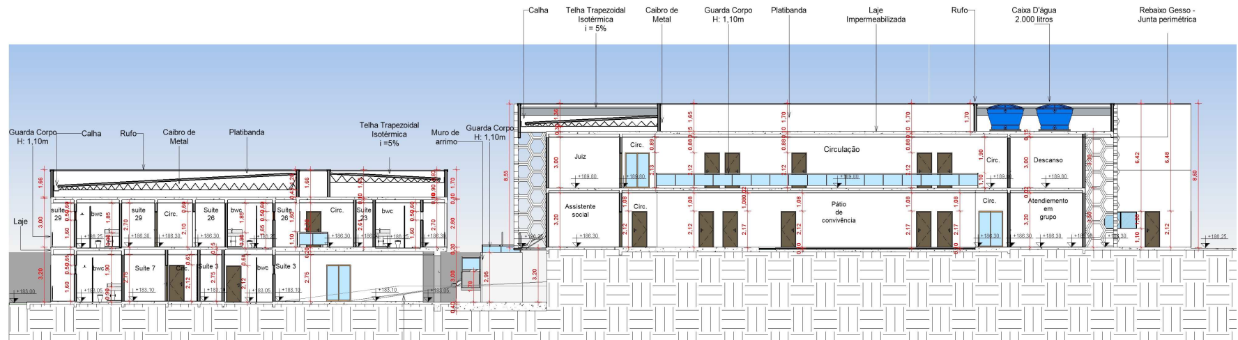
Figura 74 - Corte BB
