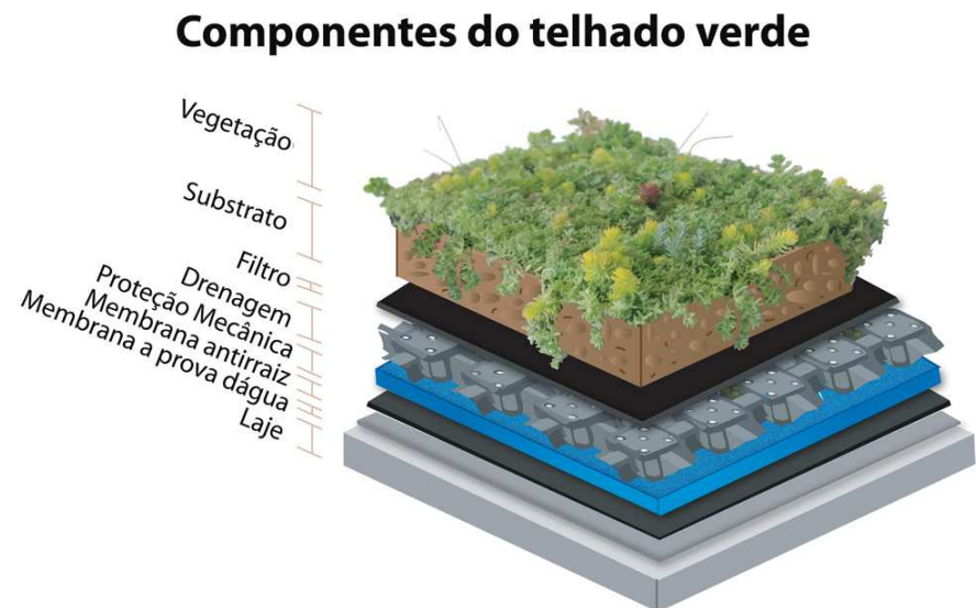
Figura 55 – Telhado Verde Intensivo
