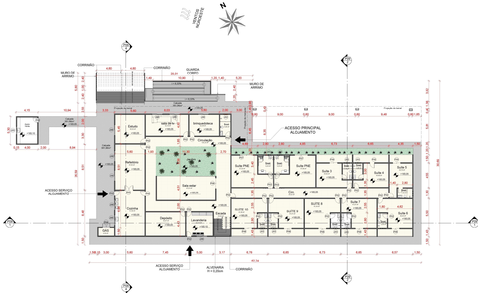
Figura 67 - Planta baixa técnica Subsolo
