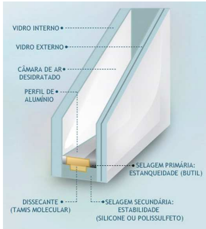
Figura 65 - Vidro Insulado
