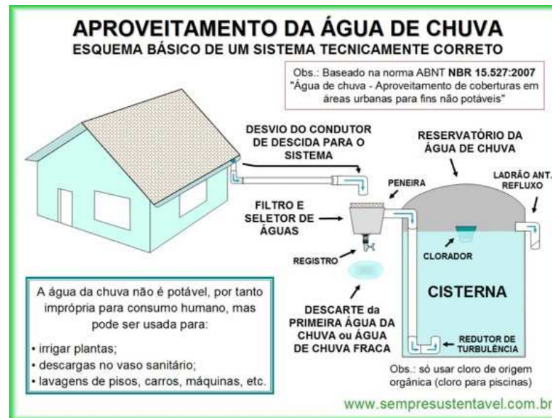
Figura 64 - Sistema de Captação de água da chuva
