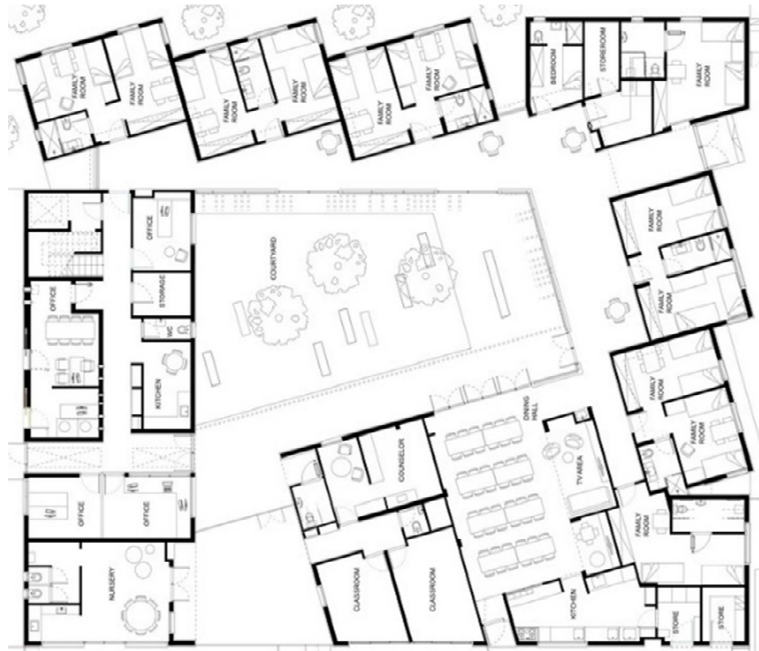
Figura 25: Planta baixa térreo
