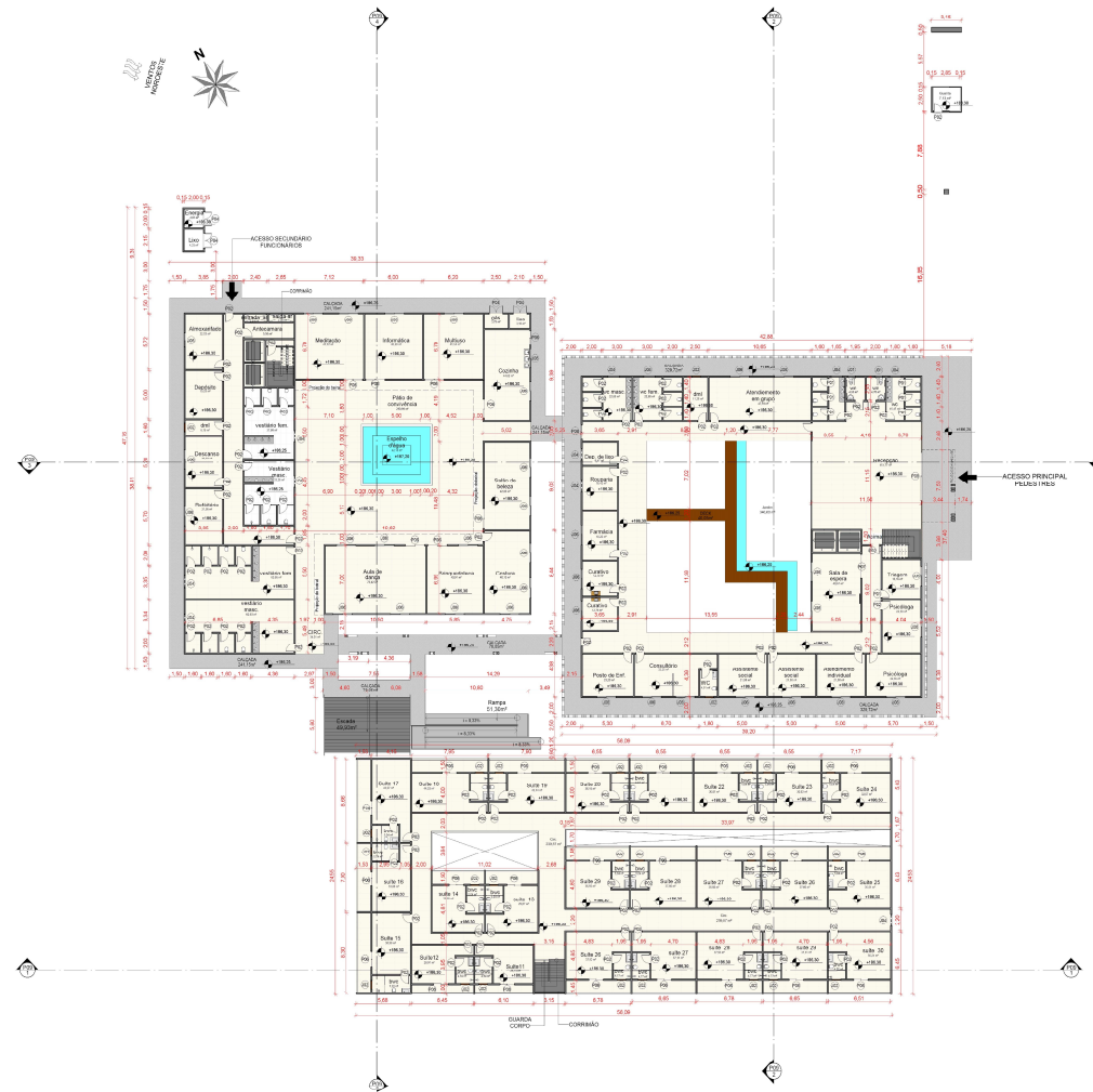
Figura 68 - Planta baixa Térreo
