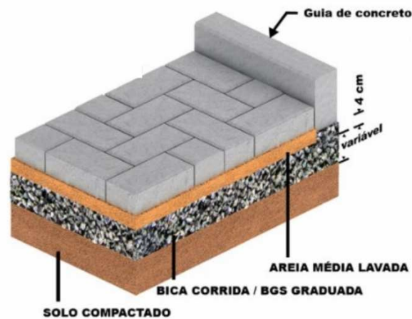
Figura 58 – Esquema de Instalação do piso
