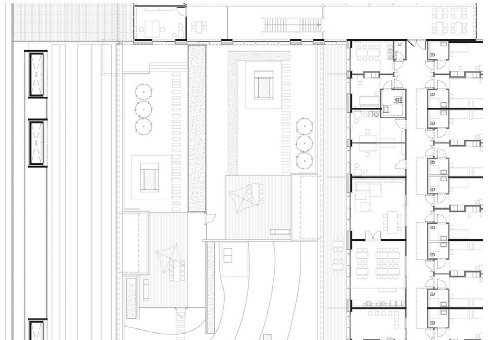
Figura 26 - Planta baixa
