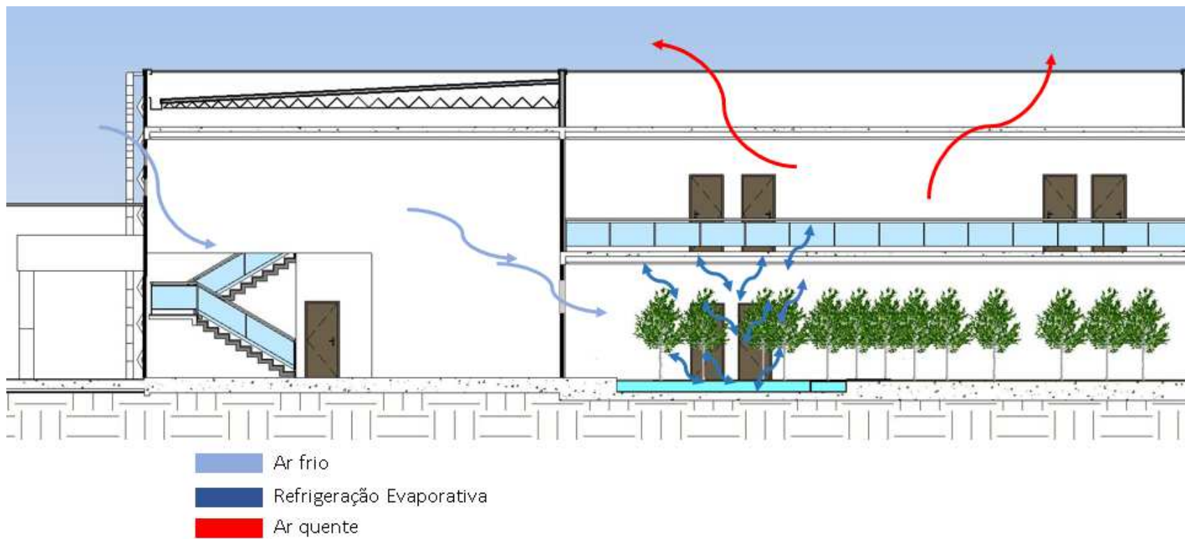
Figura 50 – Esquema de ventilação natural
