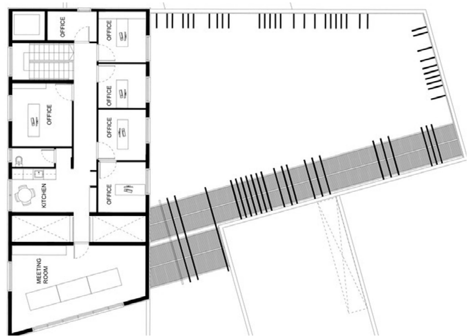
Figura 22 - Planta baixa do pavimento
